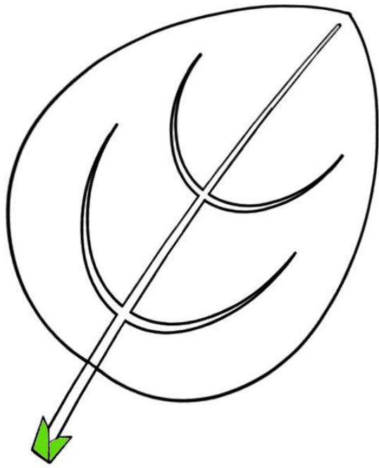
stipules
