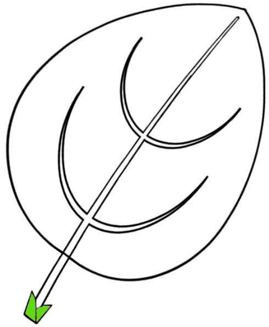
stipules
